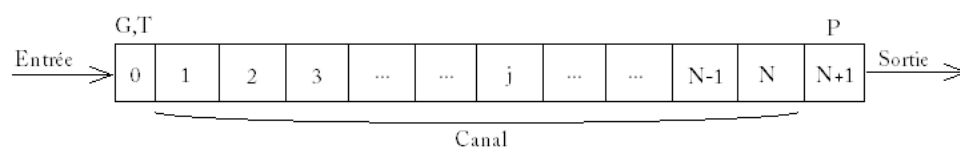
Figure 4 : Schéma du canal discrétisé.
