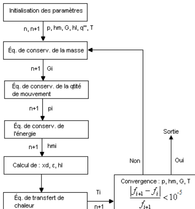
Figure 21 : Algorithme de calcul d'ARTHUR.
