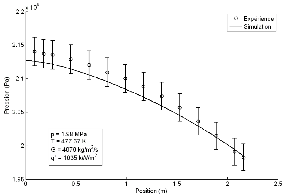
Figure 8 : Chute de pression dans l'expérience 23 (Aubé, 1996).
