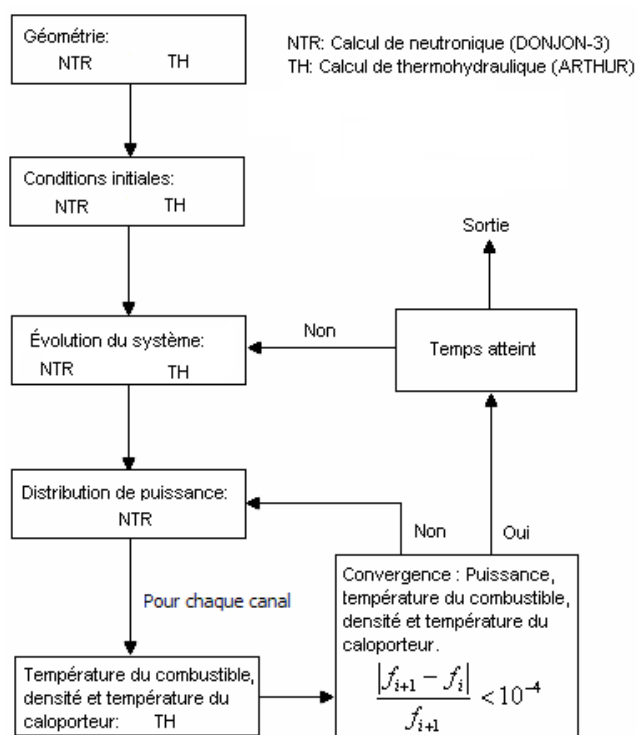
Figure 22 : Algorithme de couplage neutronique/thermohydraulique.
