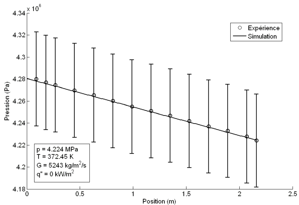
Figure 5 : Chute de pression dans l'expérience m19 (Aubé, 1996).
