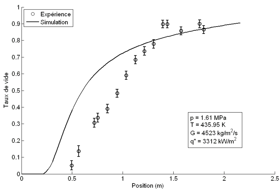
Figure 13 : Taux de vide dans l'expérience 44v (Aubé, 1996).
