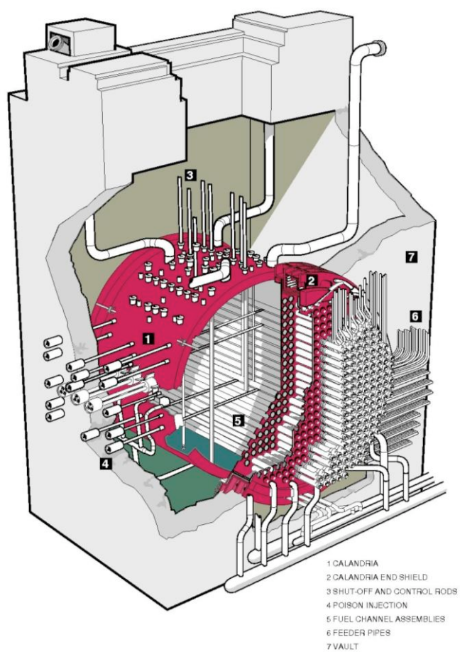
Figure 1 : Schéma de la cuve du CANDU-6.
