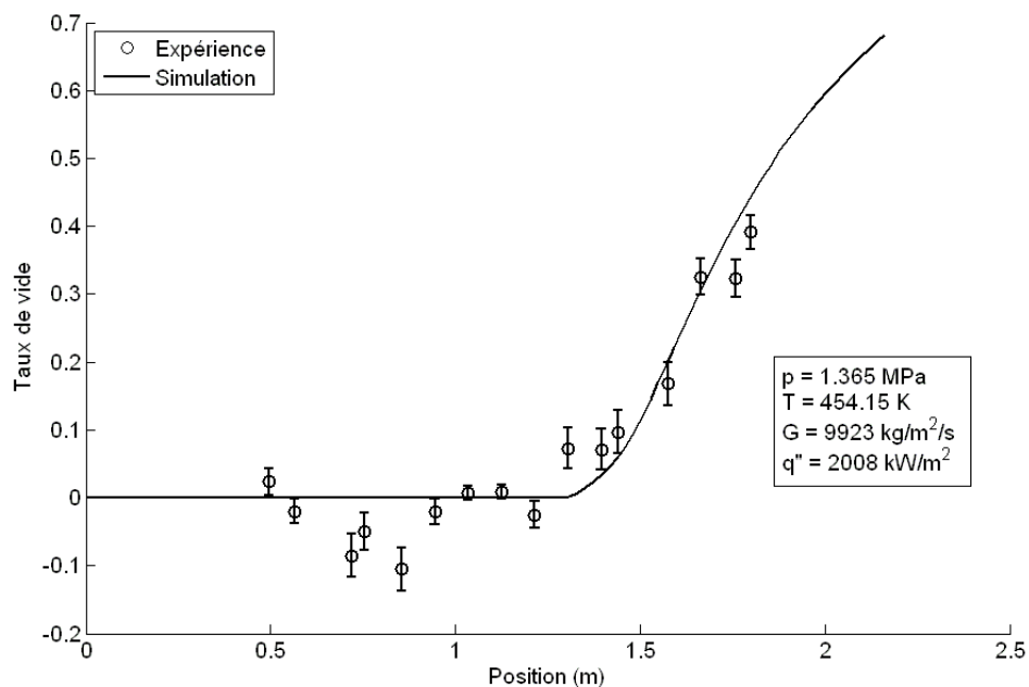
Figure 12 : Taux de vide dans l'expérience 31 (Aubé, 1996).
