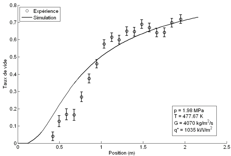
Figure 11 : Taux de vide dans l'expérience 23 (Aubé, 1996).
