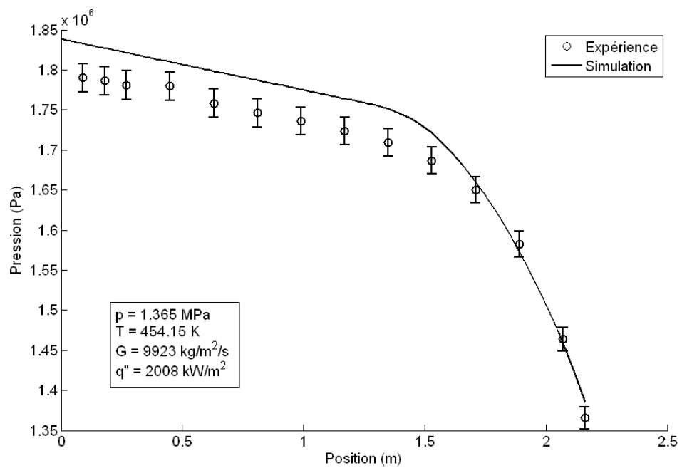
Figure 9 : Chute de pression dans l'expérience 31 (Aubé, 1996).
