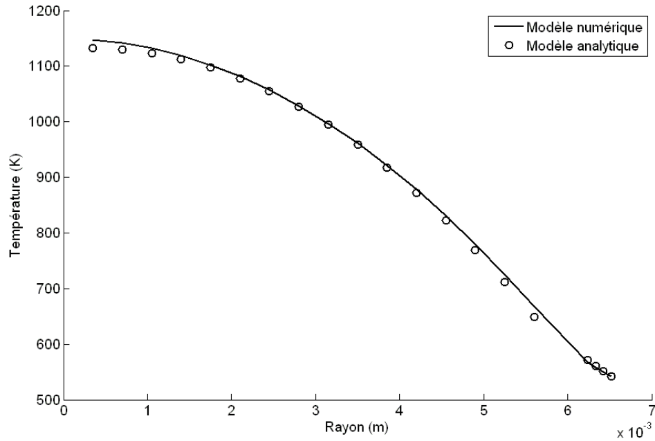
Figure 20 : Distribution de température dans un crayon.
