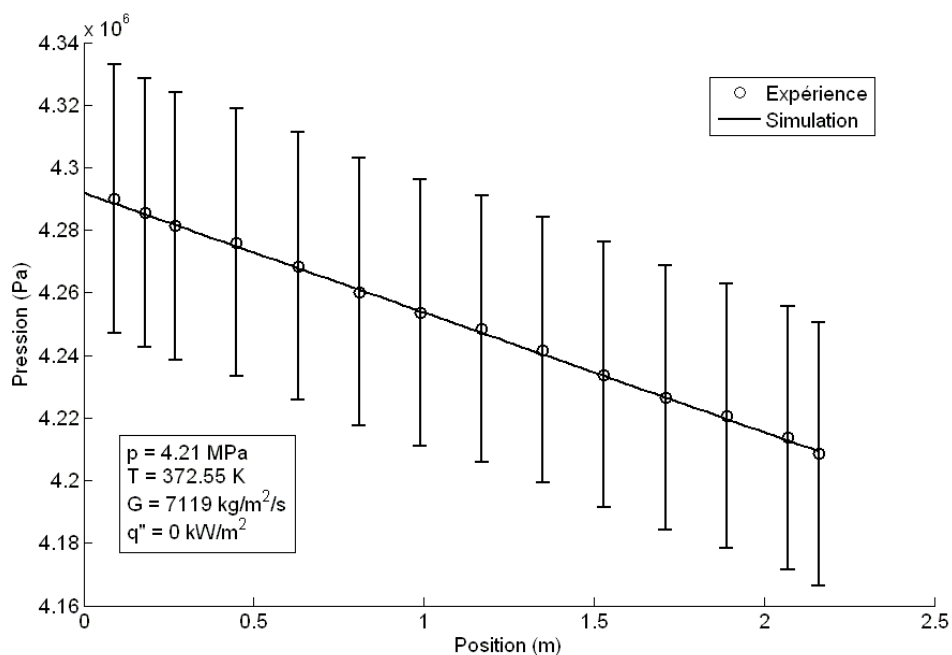
Figure 6 : Chute de pression dans l'expérience m37 (Aubé, 1996).
