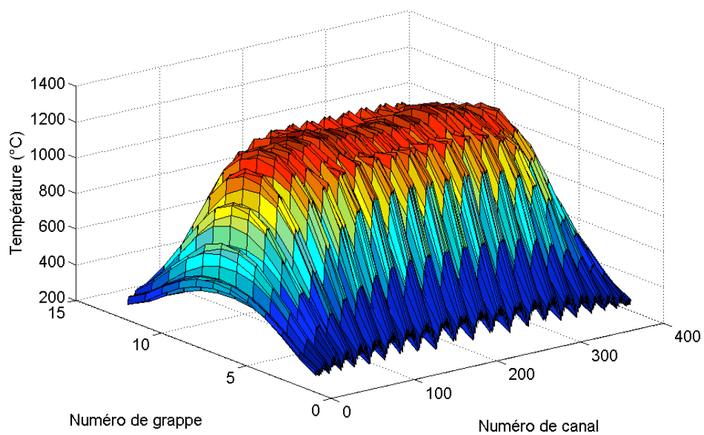
Figure 24 : Température moyenne par grappe du combustible.
