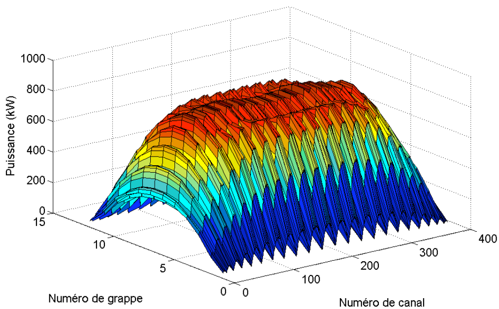
Figure 23 : Puissance moyenne par grappe.
