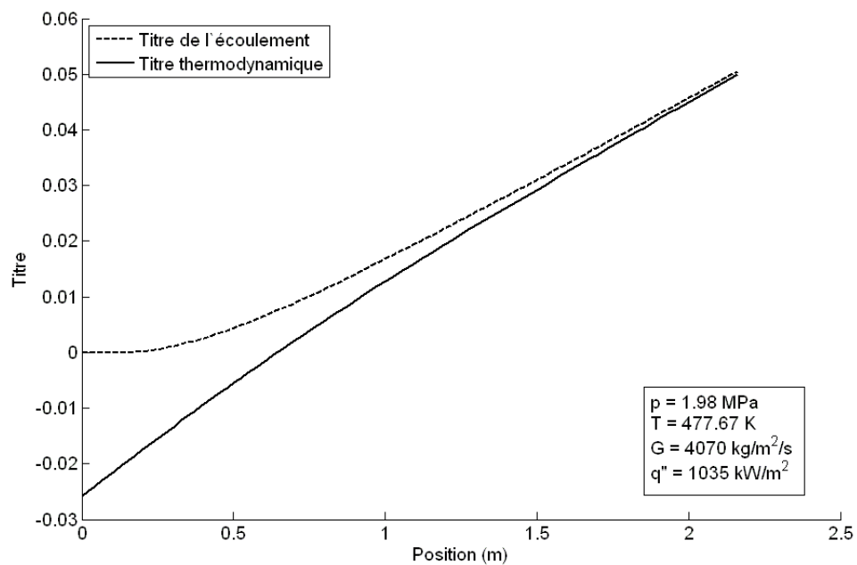
Figure 14 : Titres dans l'expérience 23 (Aubé, 1996).
