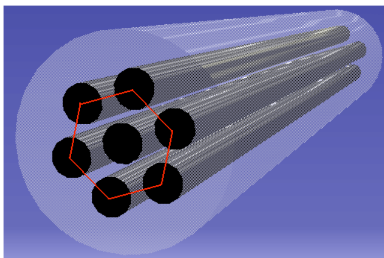
Figure 3 : Géométrie de grappe simplifiée.
