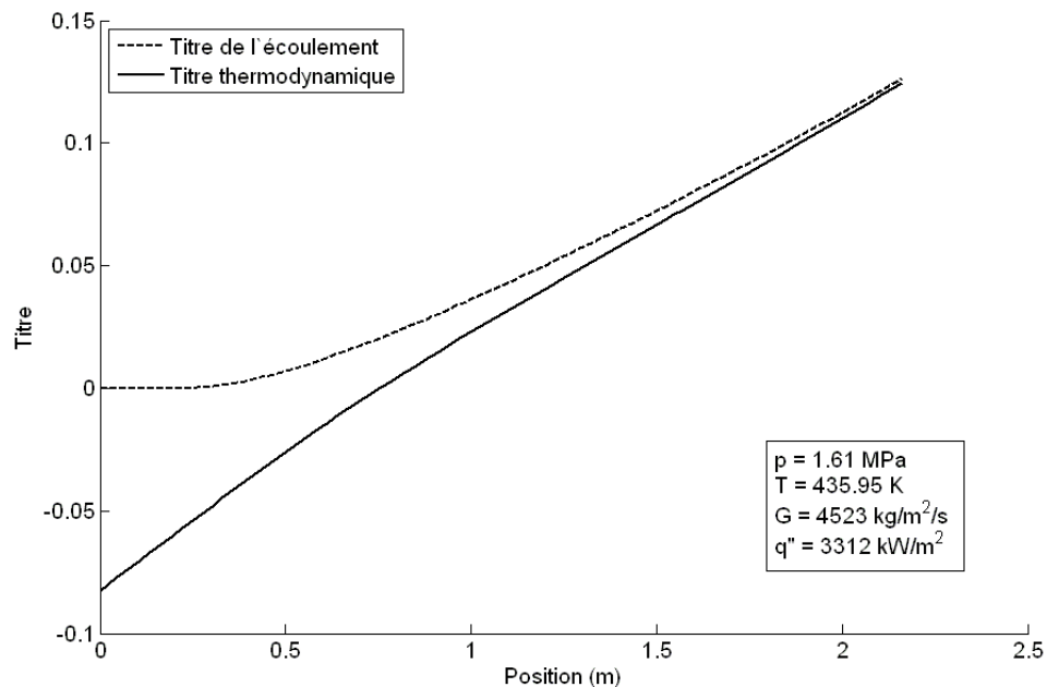
Figure 16 : Titres dans l'expérience 44v (Aubé, 1996).
