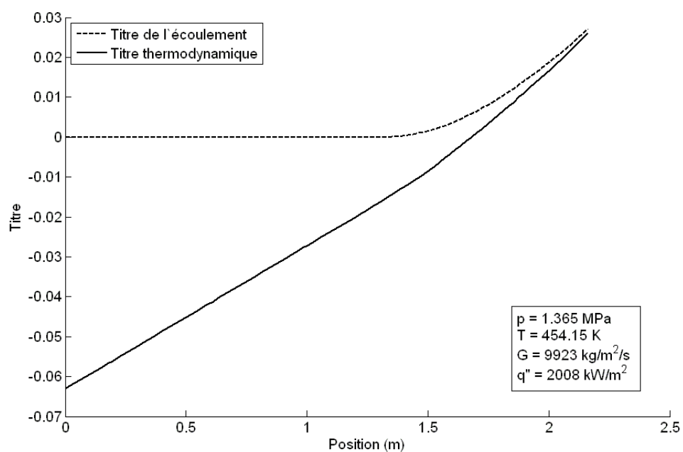
Figure 15 : Titres dans l'expérience 31 (Aubé, 1996).
