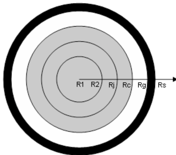
Figure 19 : Schéma du crayon.
