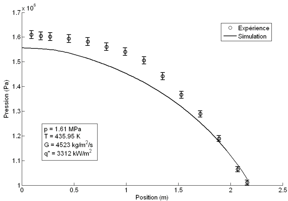
Figure 10 : Chute de pression dans l'expérience 44v (Aubé, 1996).
