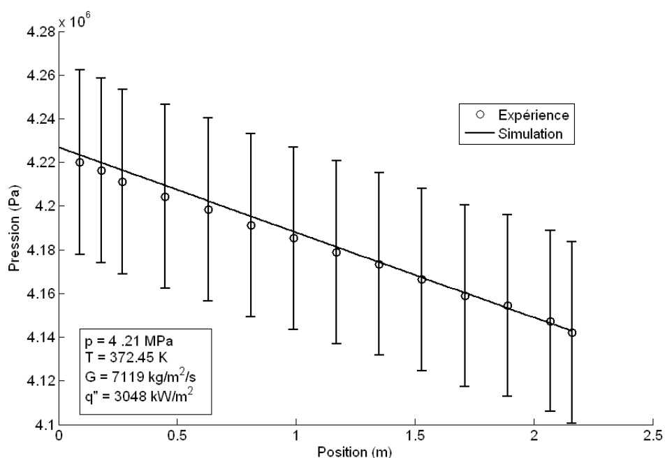
Figure 7 : Chute de pression dans l'expérience m38 (Aubé, 1996).
